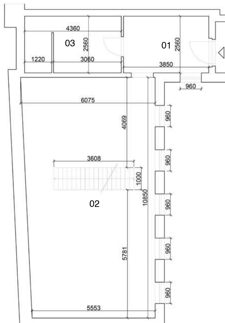
spodní podlaží main floor
